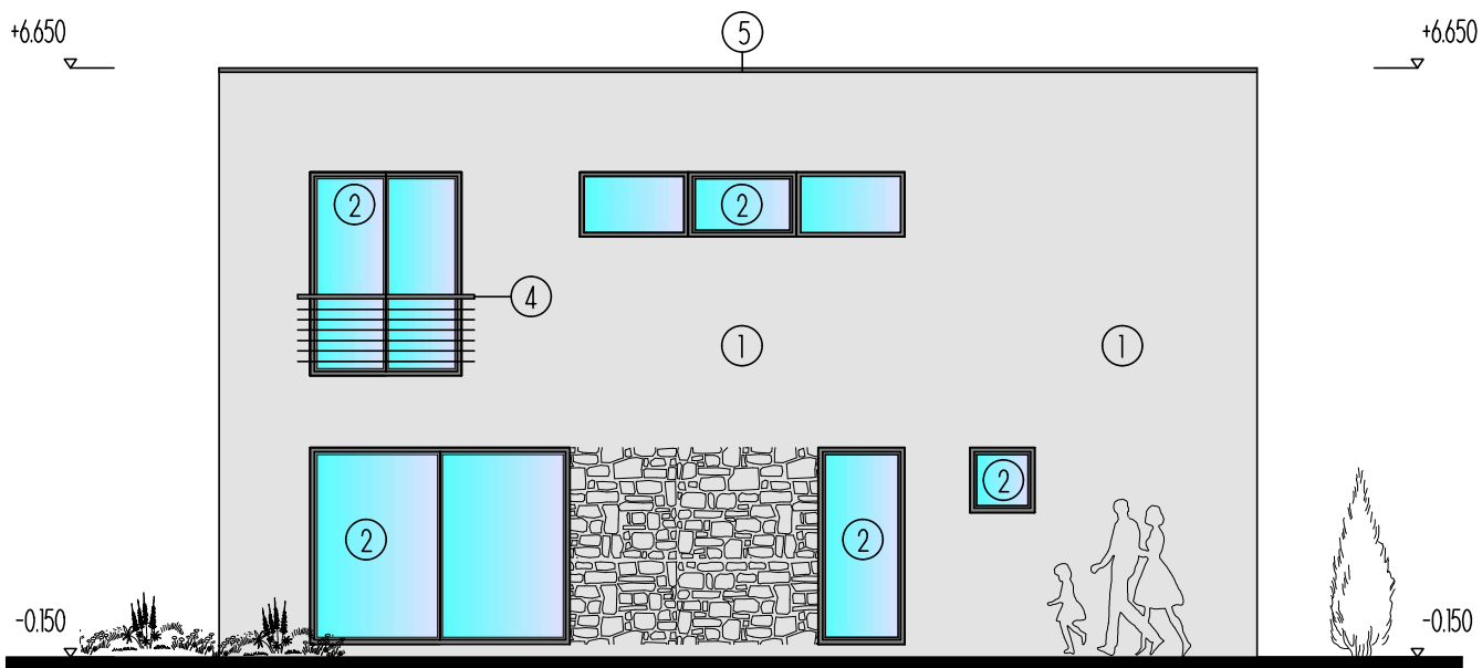
POHLÁD SEVEROVÝCHODNÝ
