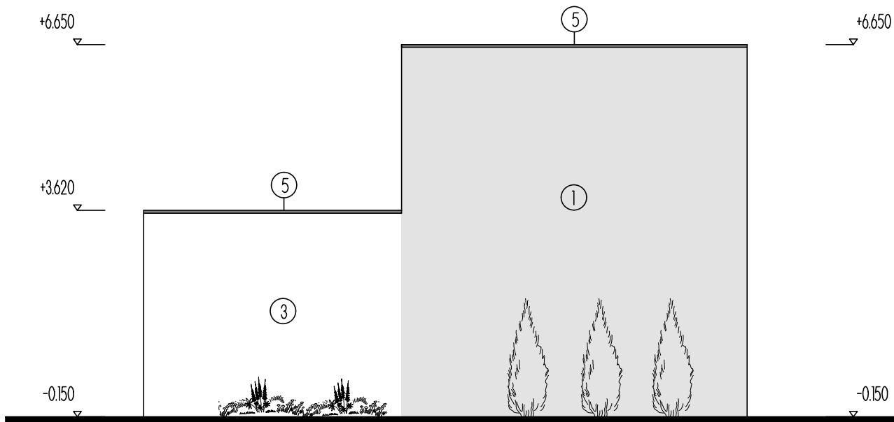
POHLÁD JUHOVÝCHODNÝ
